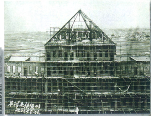
▶ 1951년 신축 중인 본관 - 본관 왼편에 직영 벽돌공장과 그 아래 제재소가 있다. 본관 비탈면의 레일은 건축자재를 옮기던 중요한 운반수단이었다. 본관 건물은 1951년 5월 26일에 상량식을 했다
